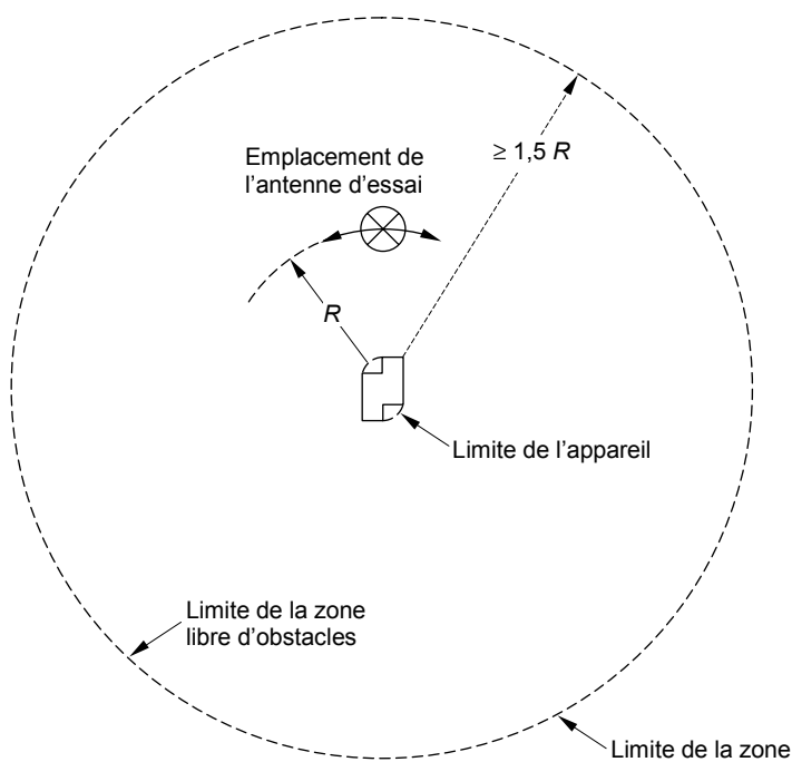
Figure 3 – Zone libre d'obstacles avec appareil en essai fixe (voir 5.3)
