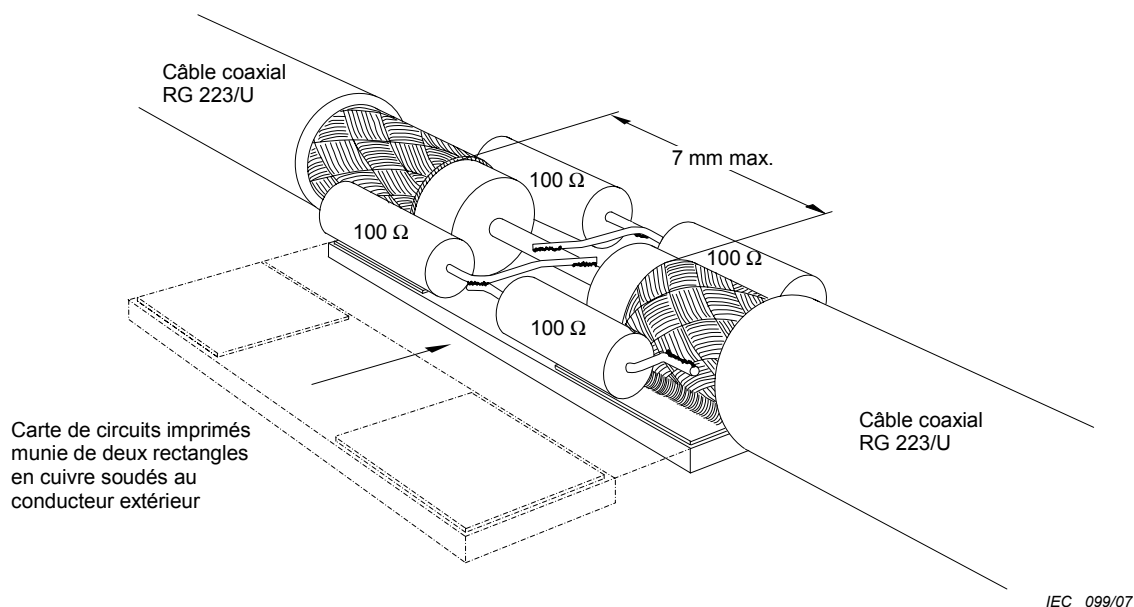
Figure C.4 – Exemple de construction de fente dont la rigidité est assurée par une plaquette de circuit imprimé
