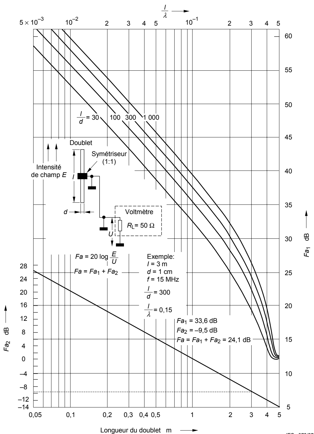
Figure 1 – Facteurs d'antenne des doublets courts pour R_L = 50 \Omega
